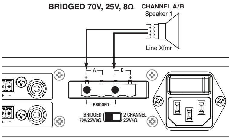
(Abbildung 1) Überbrückte Verdrahtung
