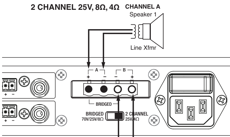
(Abbildung 2) 2-Kanal-Verdrahtung
