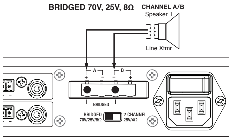
(Figura 1) Cableado con puente
