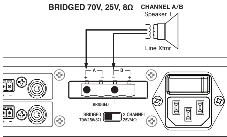
(Figure 1) Câblage ponté
