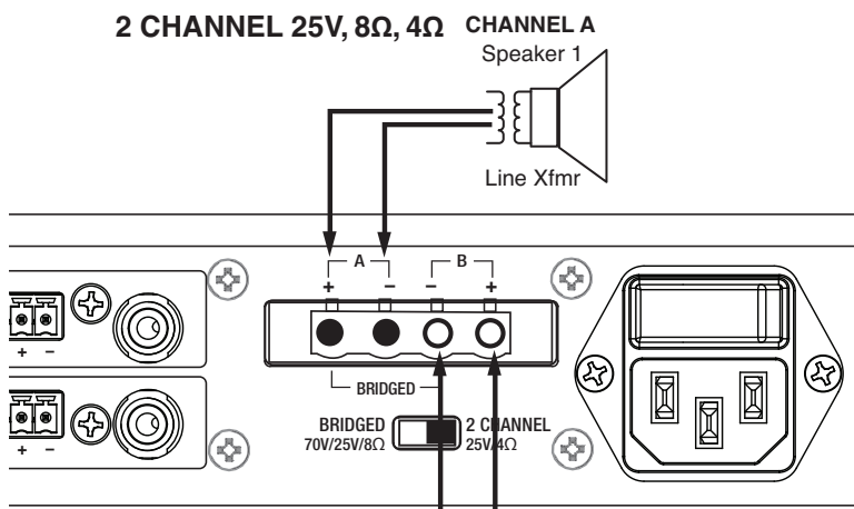
(Figura 2) Cableado de 2 canales
