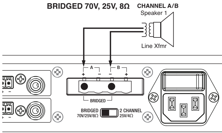
(Figuur 1) Overbruggingskabel
